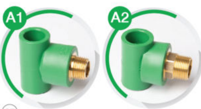
สามทางเกลียวนอกทองเหลือง พีพีอาร์ MALE TEE BRASS PP-R
